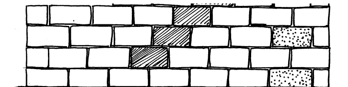
muur in "halfsteensverband"
